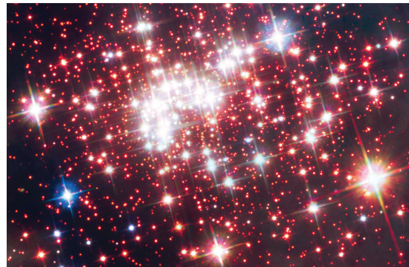
Miles de estrellas, luminosas y centelleantes, habitan en el recientemente formado cúmulo de estrellas Westerlund 2 situado en el centro de la nebulosa.
